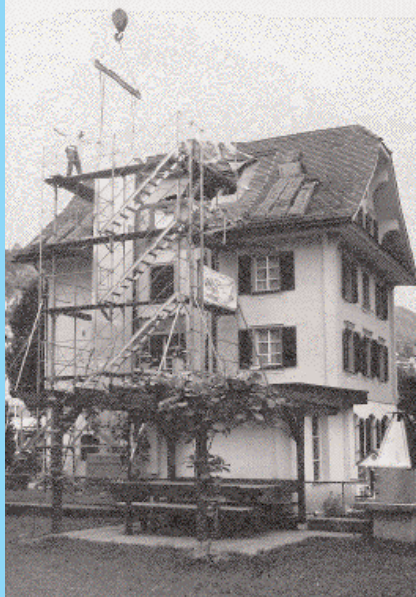
Moderne Bautechnik. Bruno Nöpfli, Chef Zimmermann, dirigiert den Kranführer mit dem vorfabrizierten Element am Haken genau in die vorbereitete Position.
